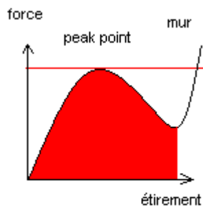
courbe de tension d'un arc compound
